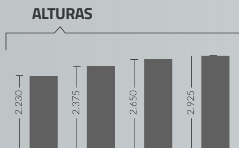
Alturas externas dos módulos. Unidade de medida em mm.
